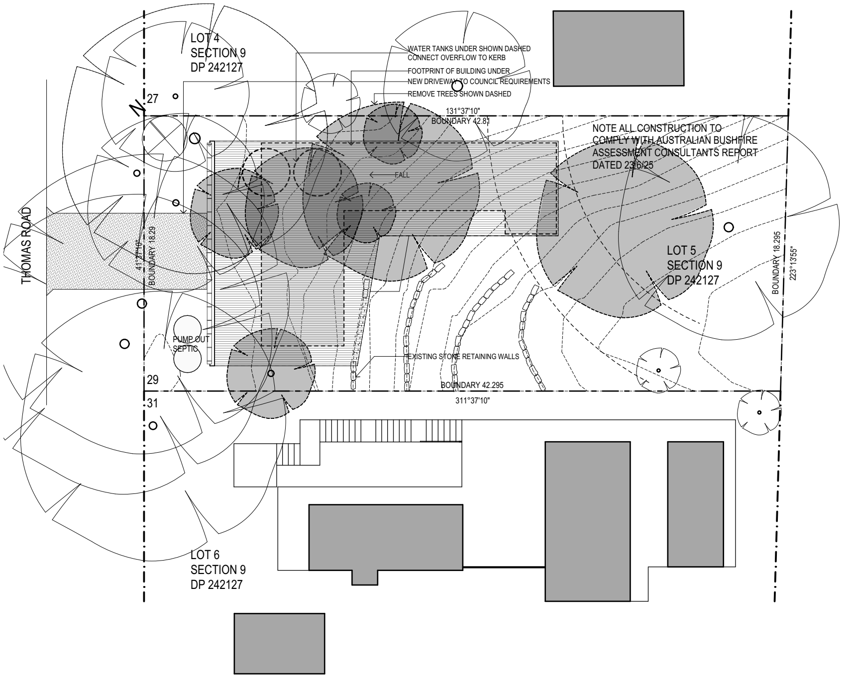
10. SITE PLAN 1:250
